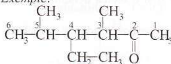
4-etil-3,5-dimetil-2-hexanonă
