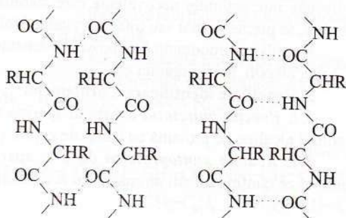
Figura 15.3.
