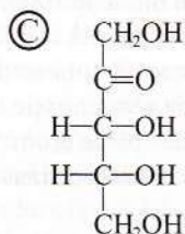
D-ribuloză
