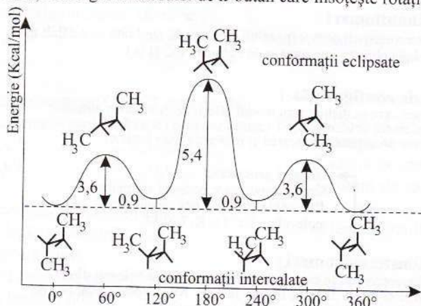
Unghiul de rotație în jurul legăturii \text{C}^2\text{—C}^3
