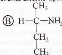
(S)-2-butanamină (S)-sec-butilamină
