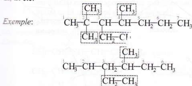
3-etil-2,2,4-trimetilheptan
