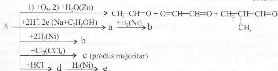
Schema 5.2.
