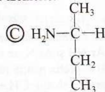
(R)-2-butanamină (R)-sec-butilamină
