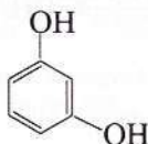
1,3-benzendiol
