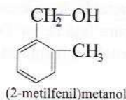
(2-metilfenil)metanol (C)
