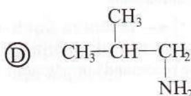
2-metil-1-propanamină izobutilamină
