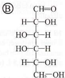
D-galactoză
