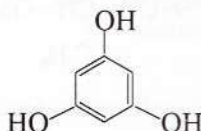
1,3,5-benzentriol
