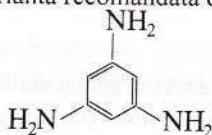
1,3,5-benzentriamină
