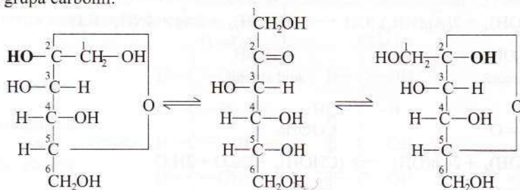
D-fructoză
