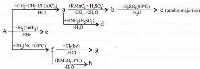
Schema 7.2.
