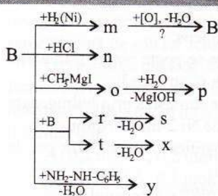
Schema 12.2.
