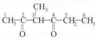
3-metil-2,4-hexandionă
