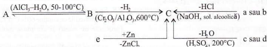
Schema 4.2.
