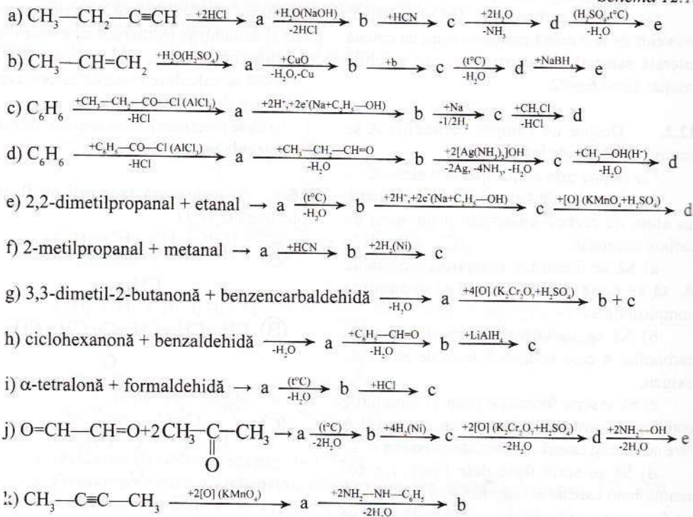
Schema 12.1.
