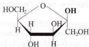
\beta -D-fructofuranoză
