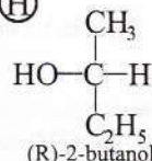
(R)-2-butanol
