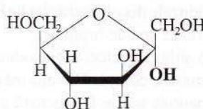
\alpha -D-fructofuranoză
