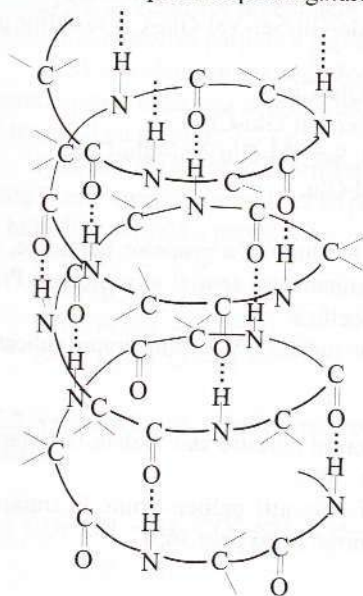
Figura 15.2.
