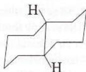
trans-decalină
