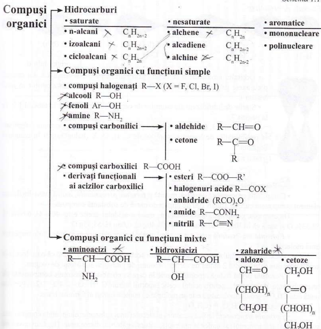
Schema 1.1.
