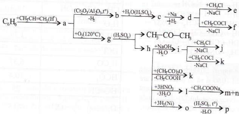
Schema 10.7.
