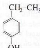
4-etilfenol (D)
