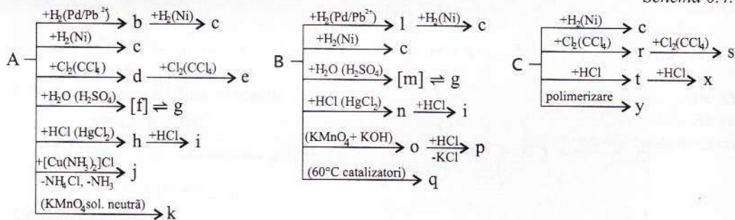
Schema 6.4.
