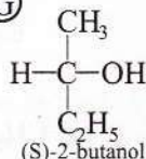
(S)-2-butanol
