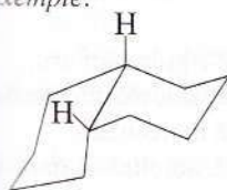
cis-decalină
